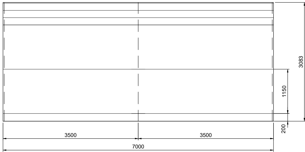
2 LEFT ELEVATION 3 SCALE: 1:50
