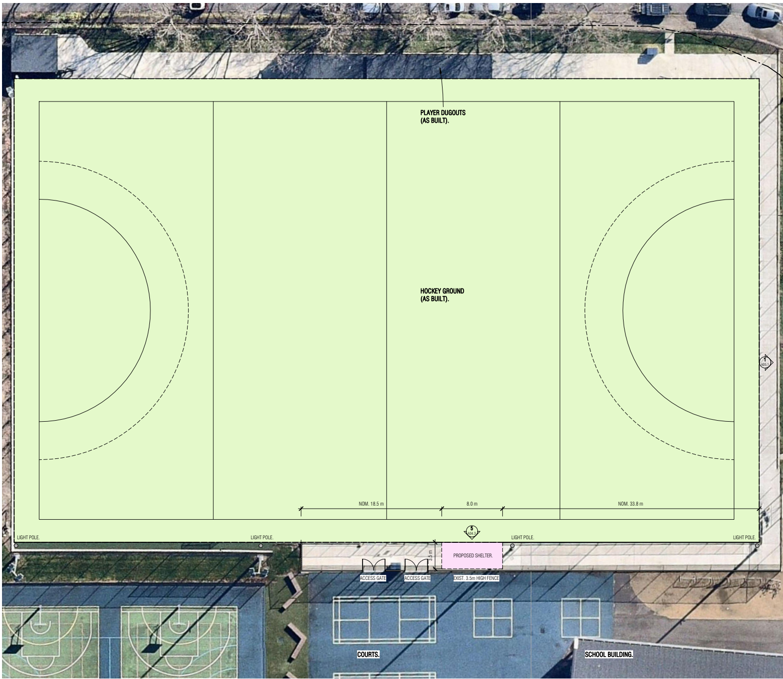
1 Site Plan - Shelter 1:250
