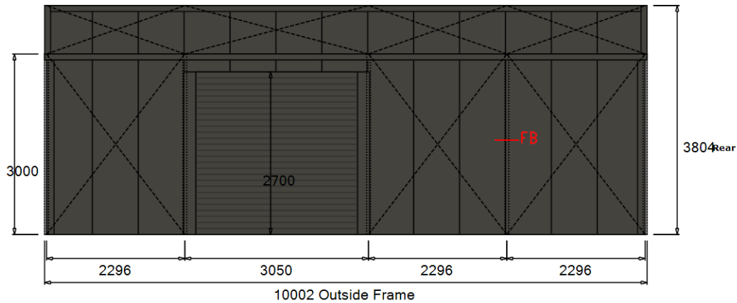
Right Elevation
