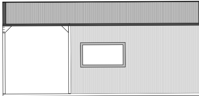
SE Ext Elevation
