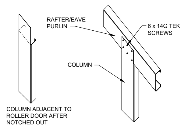
F TOP HAT CONNECTION
