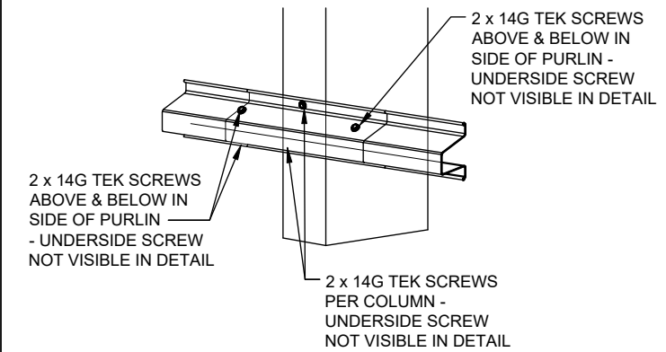
F TOP HAT CONNECTION
