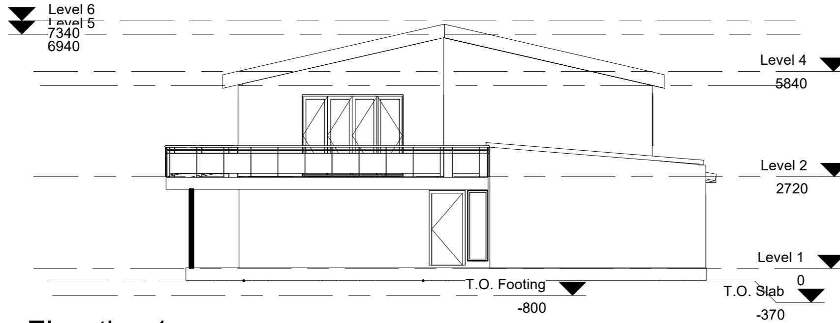
2 Elevation 1 - a 1 : 100
