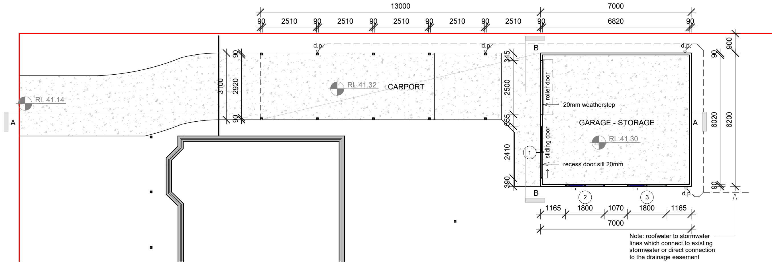
1 GARAGE - CARPORT PLAN 1 : 100
