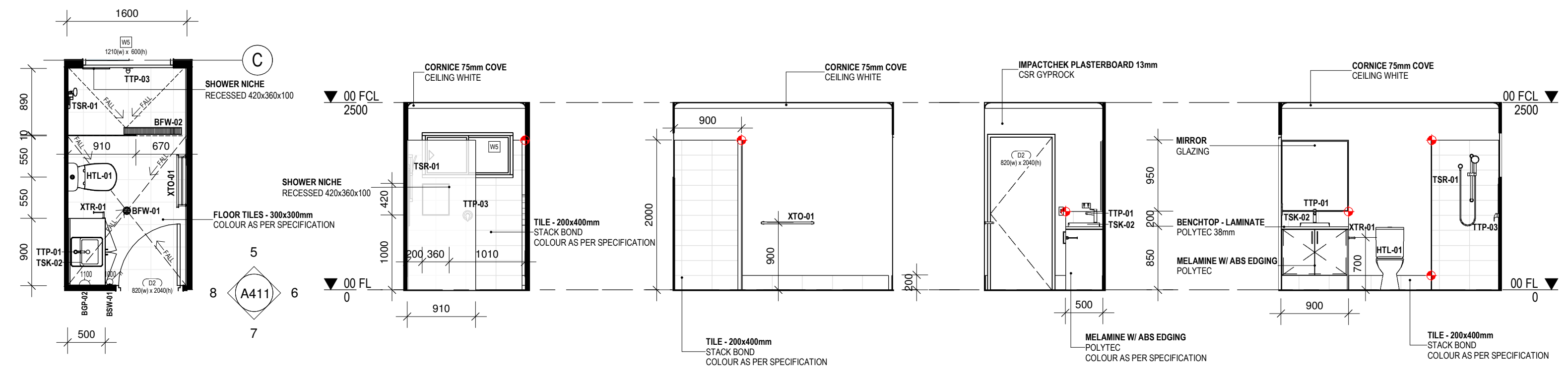
C BATH 2 PLAN 1 : 50
