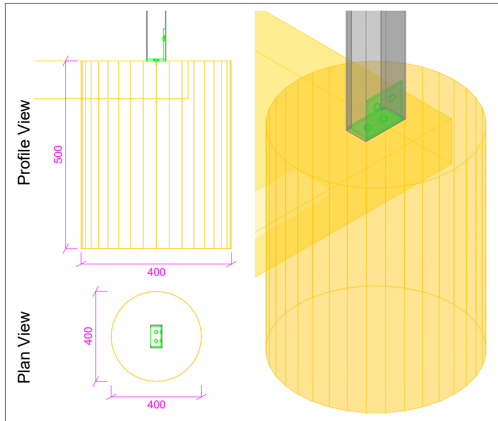
Footing: F1 (x8)
