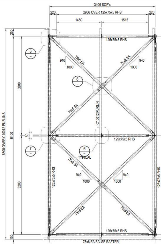
PLAN SCALE 1:25 001
