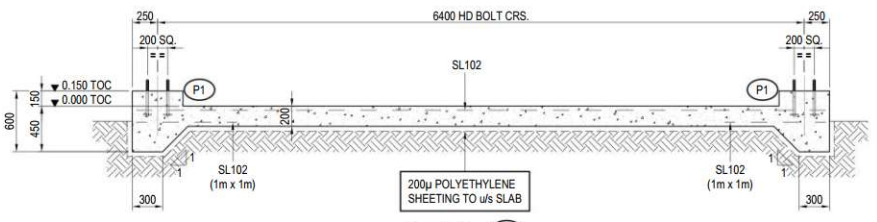
SECTION A-A SCALE 1:25
