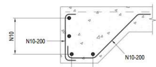
EDGE BEAM (EB) SCALE 1:10
