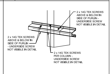
G TOP HAT CONNECTION
