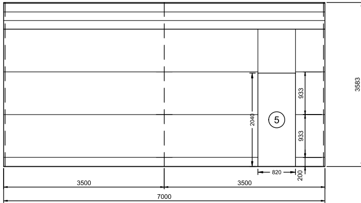
2 LEFT ELEVATION 4 SCALE: 1:50
