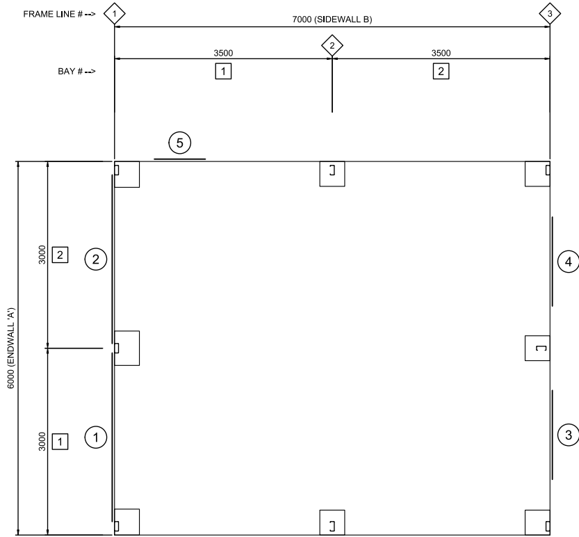
1 FLOOR PLAN 5 SCALE: 1:50
