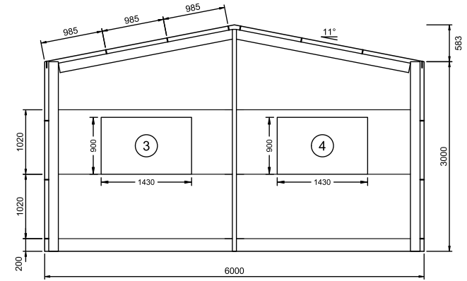
3 REAR ELEVATION 4 SCALE: 1:50 FRAME #3
