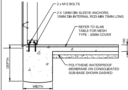
Y SLAB DETAIL
