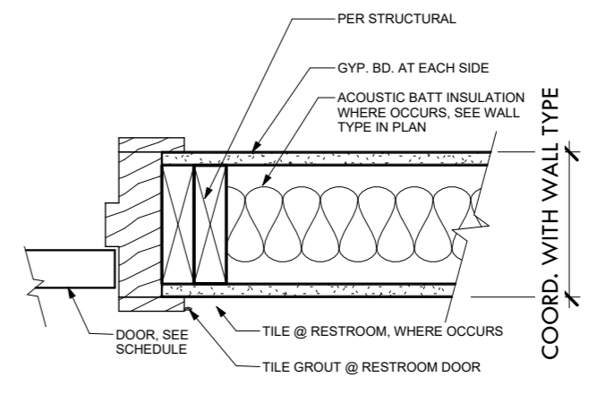
INTERIOR DOOR JAMB @ WOOD STUD
