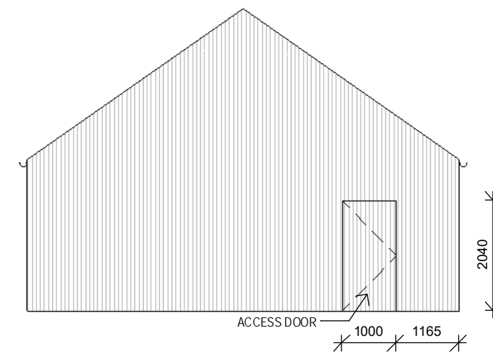
Elevation 4 1 : 100
